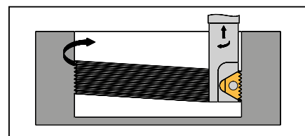
Попутное фрезерование
