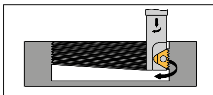
Встречное фрезерование
