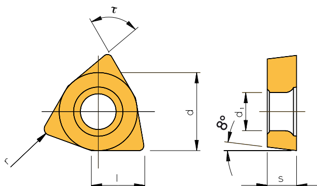
Сменные пластины / Indexable inserts / Plaquettes amovibles
